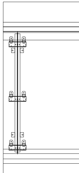
WIDOK
