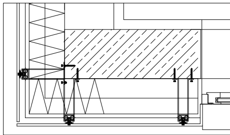
PRZEKRÓJ POPRZECZNY
