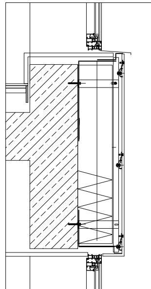
PRZEKRÓJ PODŁUŻNY
